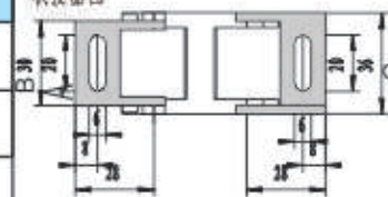
SU1825E 连接器图
