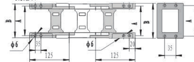
联接器图
