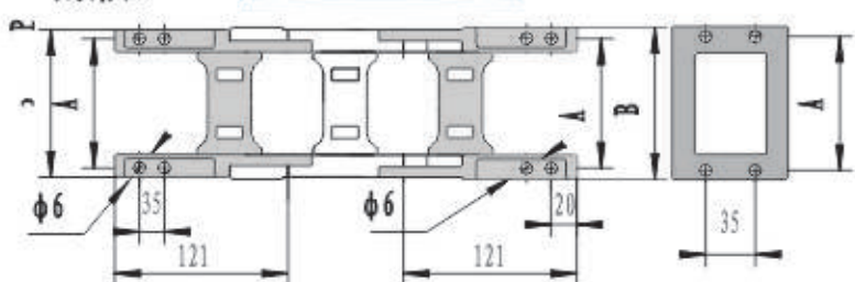
联接器图
