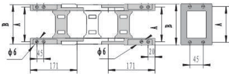
连接器图
